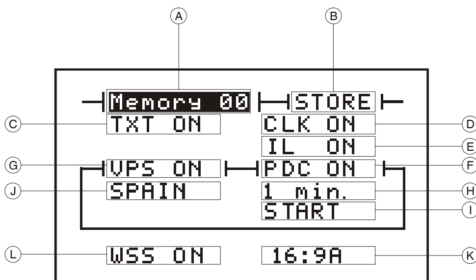
Figure 6.- Exemple d'affichage du menu de configuration TXT-VPS
