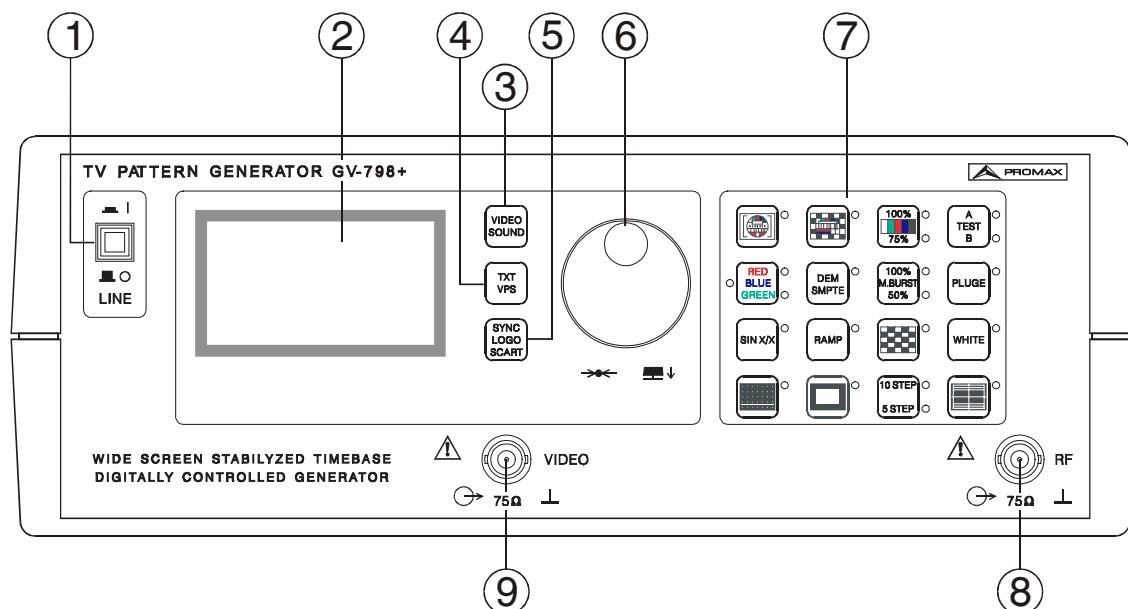
Figura 2.- Panel frontal
