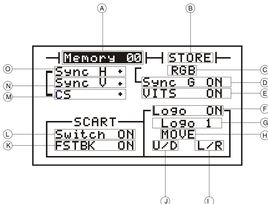
Figura 7.- Ejemplo de display del menú de configuración SYNC-LOGO-SCART
