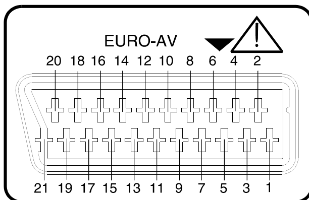
Figura 9.- Euroconector
