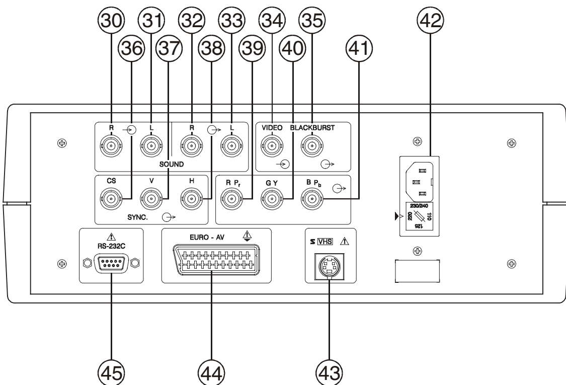
Figura 3.- Panel posterior
