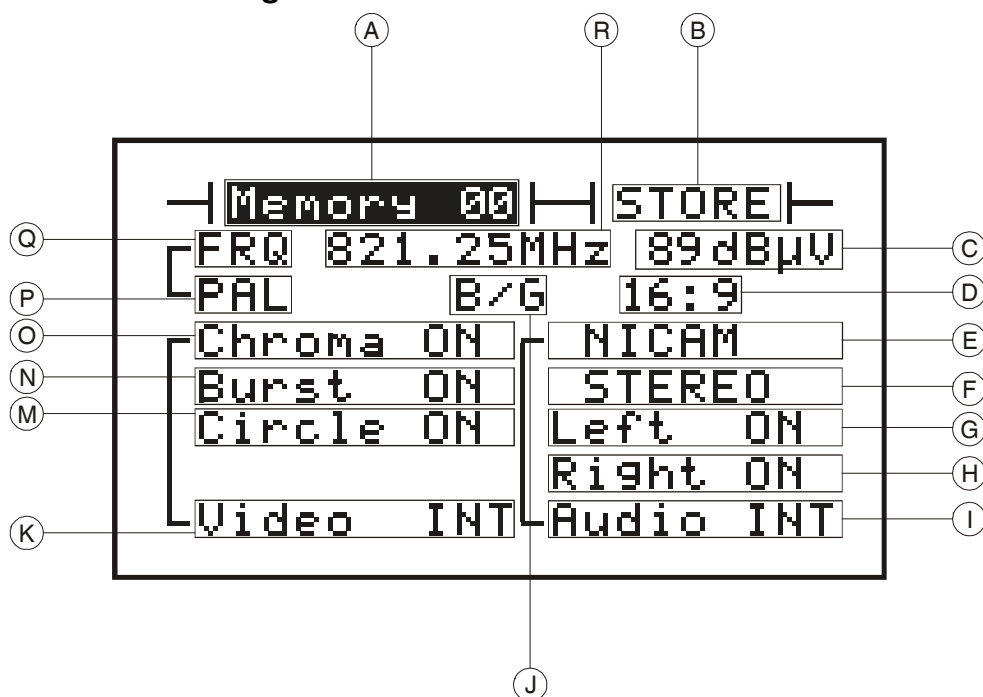
Figura 5.- Ejemplo de display del menú de configuración VIDEO-SOUND
