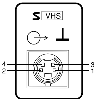
Figura 8.- Conector S-VHS
