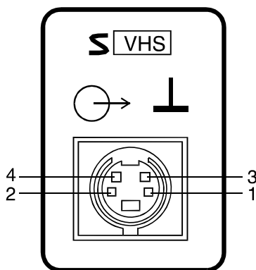
Figure 8.- Connecteur S-VHS
