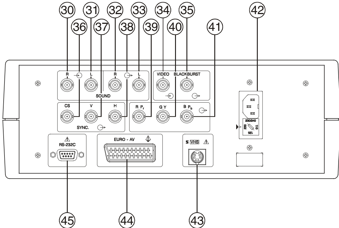
Figure 3.- Panneau arrière
