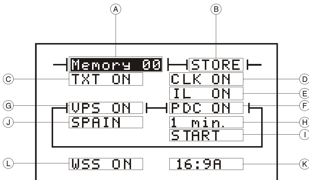
Figura 6.- Ejemplo de display del menú de configuración TXT-VPS
