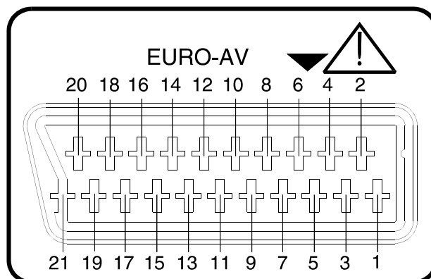
Figure 9.- Euroconnecteur
