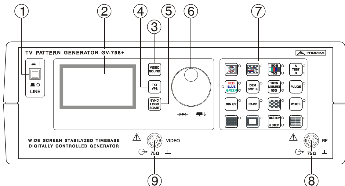
Figure 2.- Panneau avant
